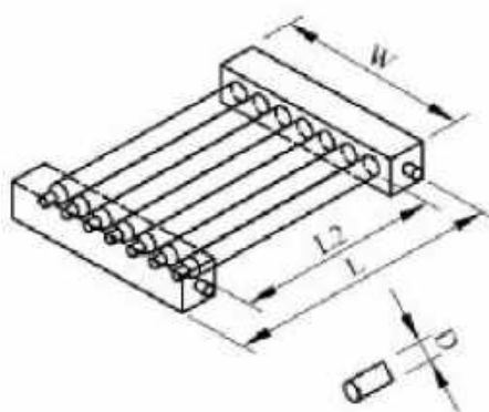
图 C.0.2 真空管集热器示意图(D—真空管直径)
