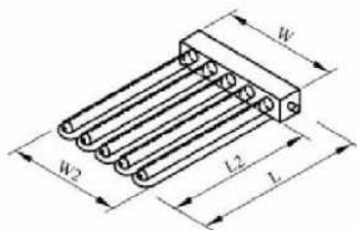
图 C.0.4 背面带反射板真空管集热器示意图
