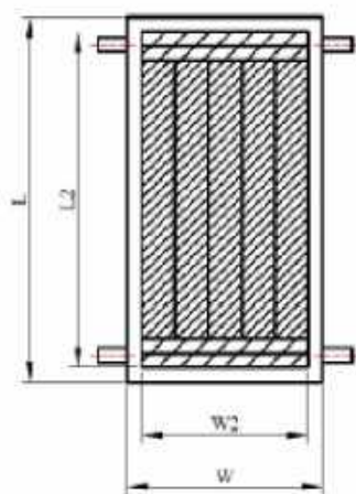
图 C.0.1 平板集热器示意图
